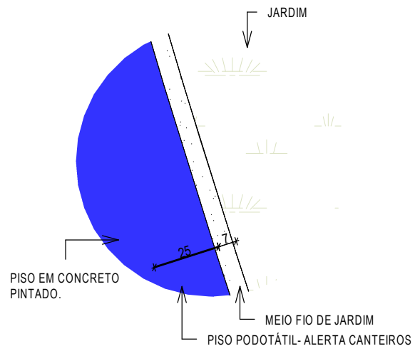
2 DETALHE DO MEIO FIO DE JARDIM 1 : 20
