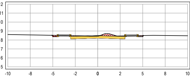
SEÇÃO TRANSVERSAL: 27+0
