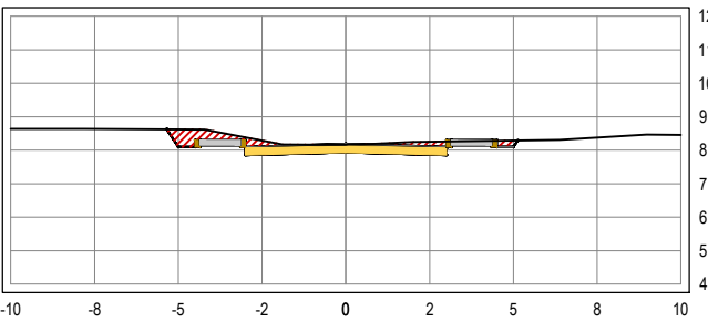
SEÇÃO TRANSVERSAL: 28+10
