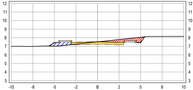
SEÇÃO TRANSVERSAL: 32+11
