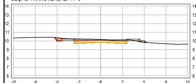
SEÇÃO TRANSVERSAL: 11+0
