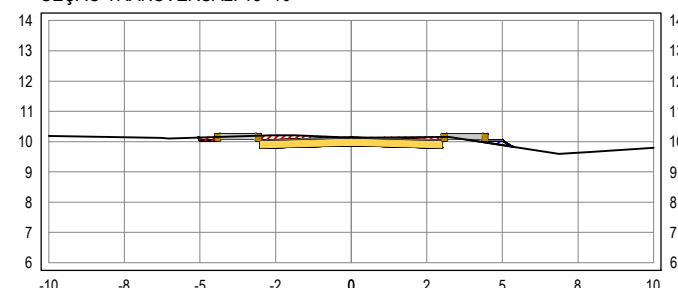
SEÇÃO TRANSVERSAL: 15+10
