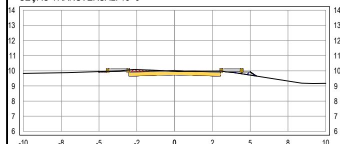
SEÇÃO TRANSVERSAL: 15+0
