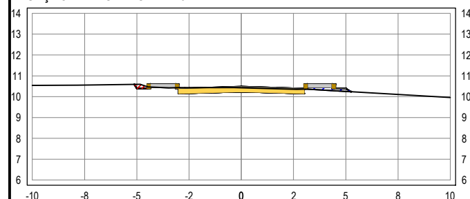
SEÇÃO TRANSVERSAL: 9+0
