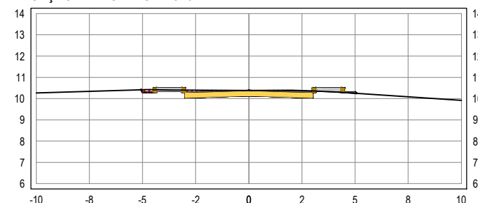
SEÇÃO TRANSVERSAL: 10+0
