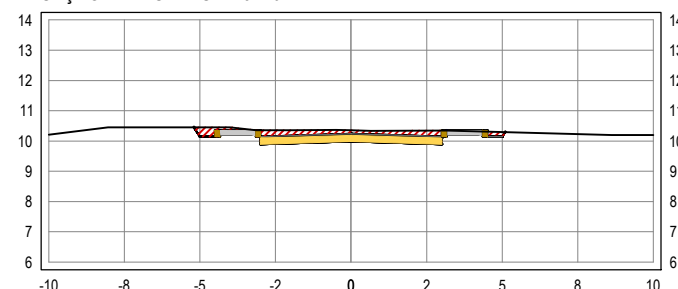
SEÇÃO TRANSVERSAL: 11+10
