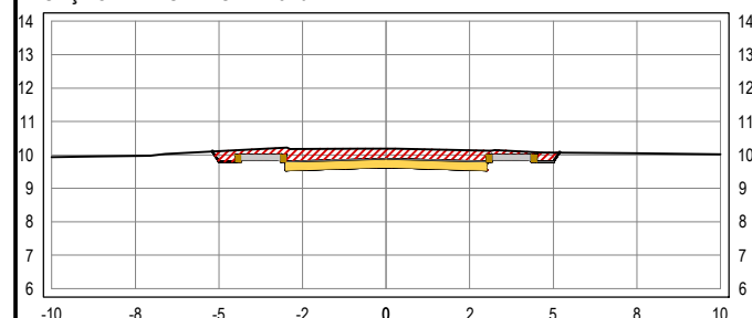
SEÇÃO TRANSVERSAL: 13+0
