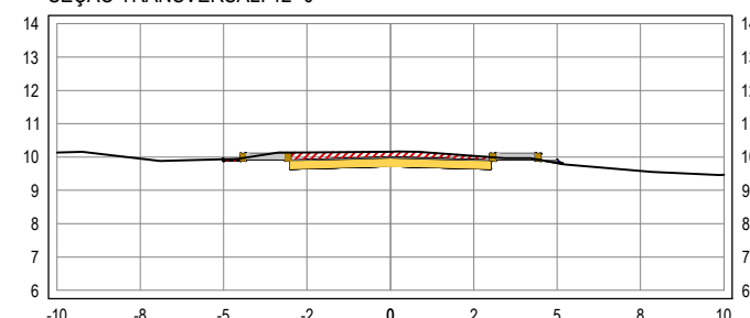
SEÇÃO TRANSVERSAL: 12+0
