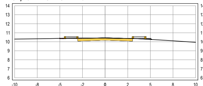
SEÇÃO TRANSVERSAL: 9+10
