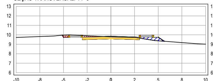
SEÇÃO TRANSVERSAL: 14+0
