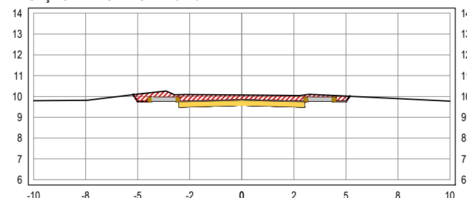
SEÇÃO TRANSVERSAL: 13+10
