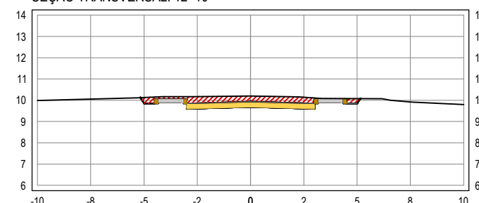
SEÇÃO TRANSVERSAL: 12+10
