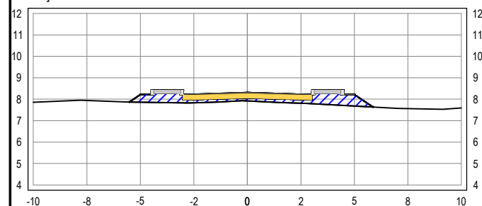
SEÇÃO TRANSVERSAL: 16+10
