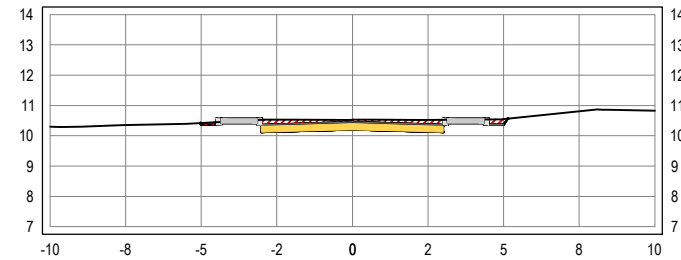
SEÇÃO TRANSVERSAL: 11+10
