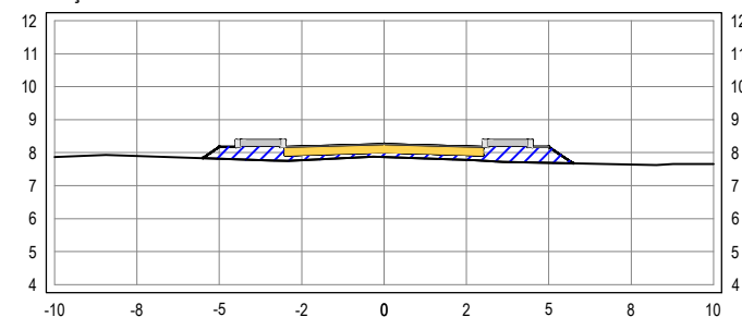
SEÇÃO TRANSVERSAL: 17+0
