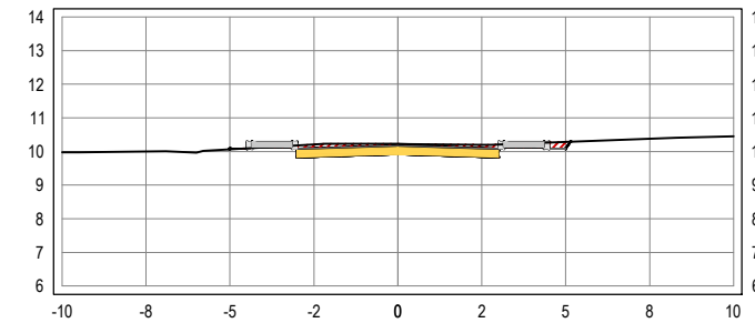
SEÇÃO TRANSVERSAL: 12+0
