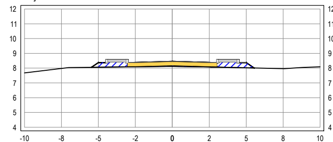
SEÇÃO TRANSVERSAL: 15+0
