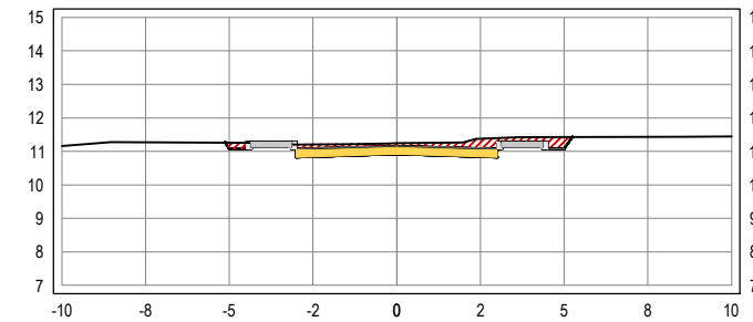
SEÇÃO TRANSVERSAL: 10+0
