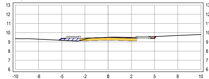
SEÇÃO TRANSVERSAL: 13+0
