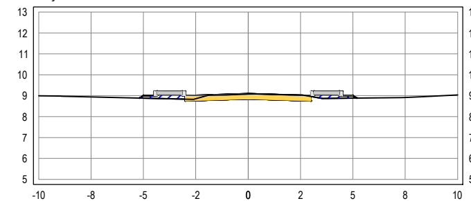
SEÇÃO TRANSVERSAL: 13+10
