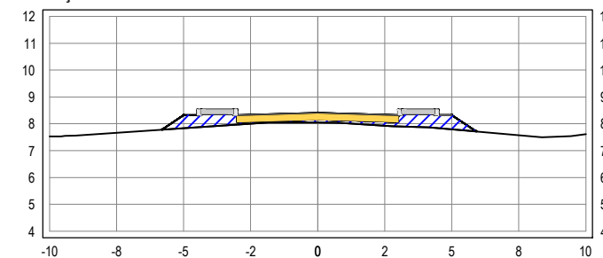
SEÇÃO TRANSVERSAL: 15+10
