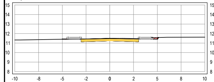
SEÇÃO TRANSVERSAL: 9+0
