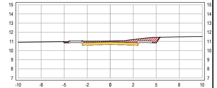
SEÇÃO TRANSVERSAL: 10+10
