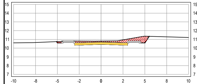
SEÇÃO TRANSVERSAL: 11+0
