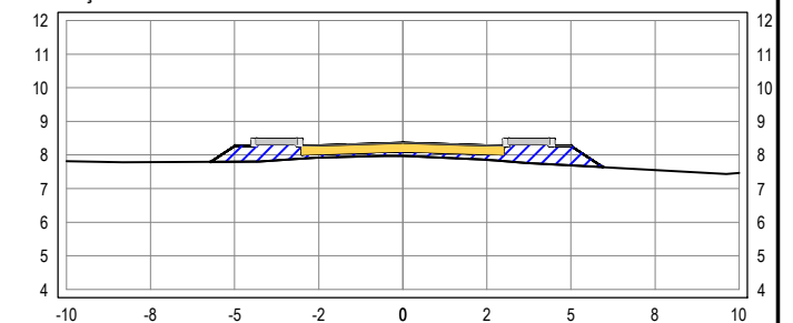
SEÇÃO TRANSVERSAL: 16+0
